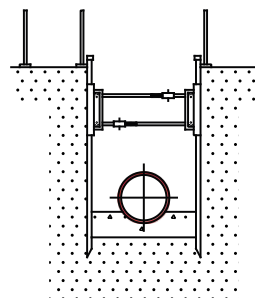
SECCION B-B
